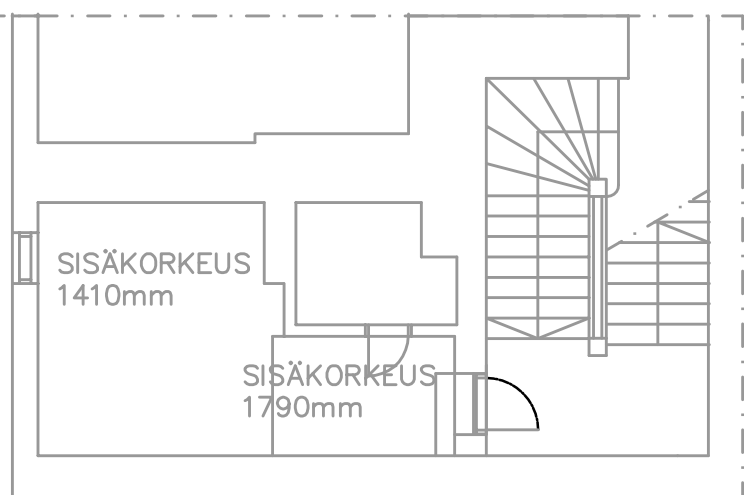
1 1/2-KERROS
